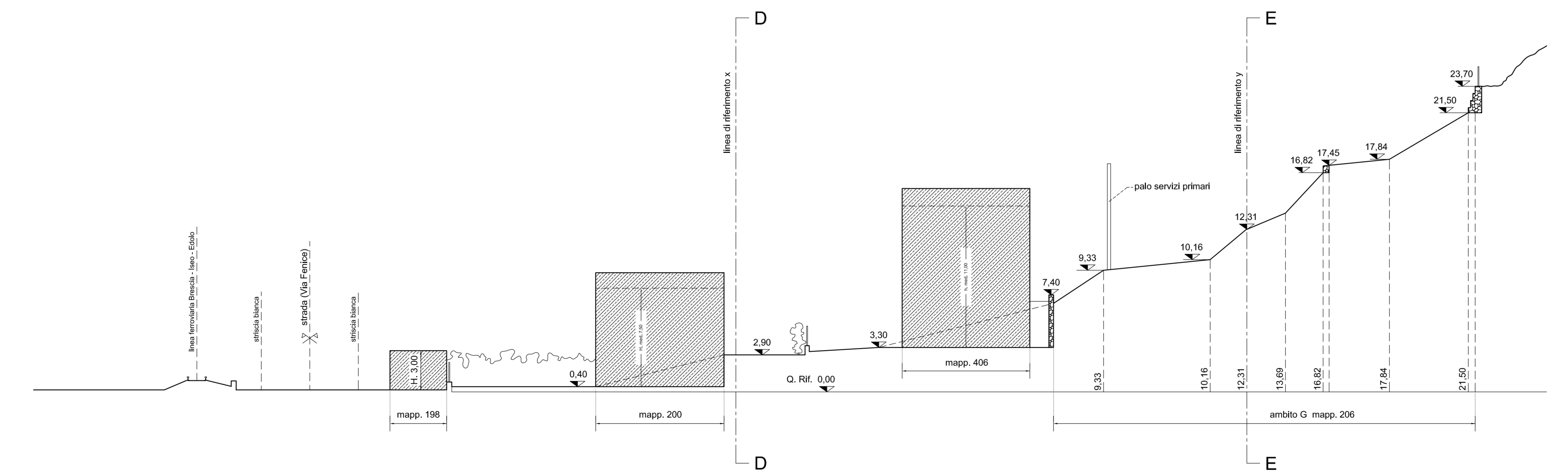
SEZIONE C-C scala 1:200
