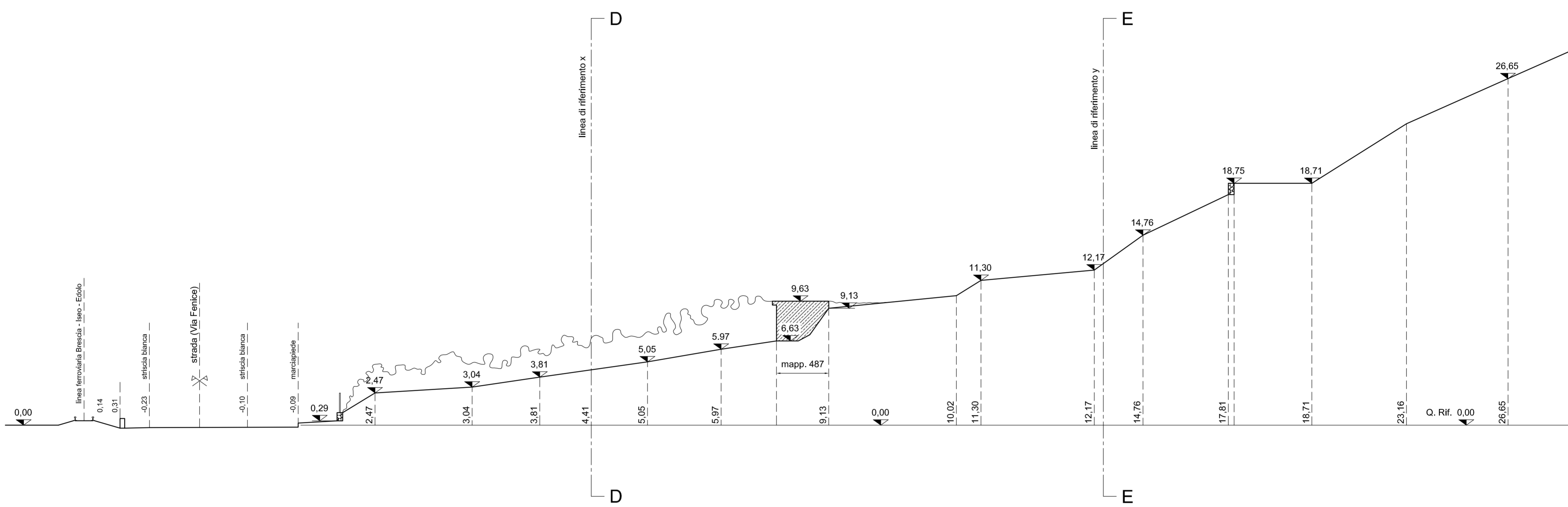
SEZIONE B-B scala 1:200
