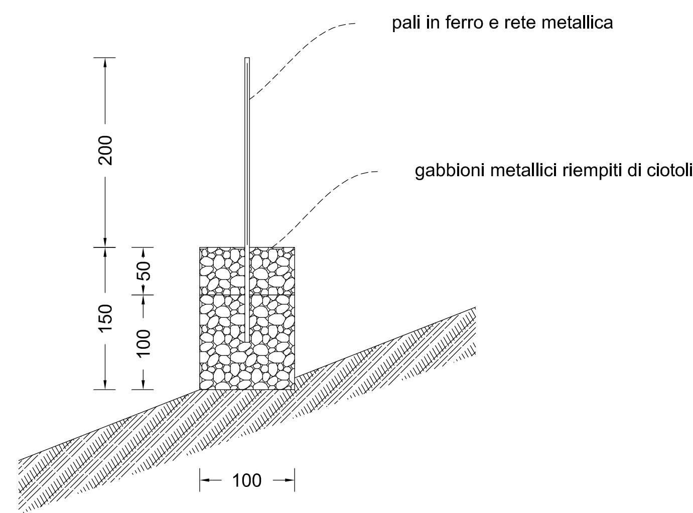
SEZIONE TIPO 1:40
