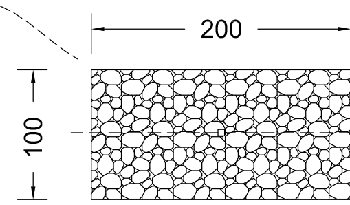
PIANTA 1:40
