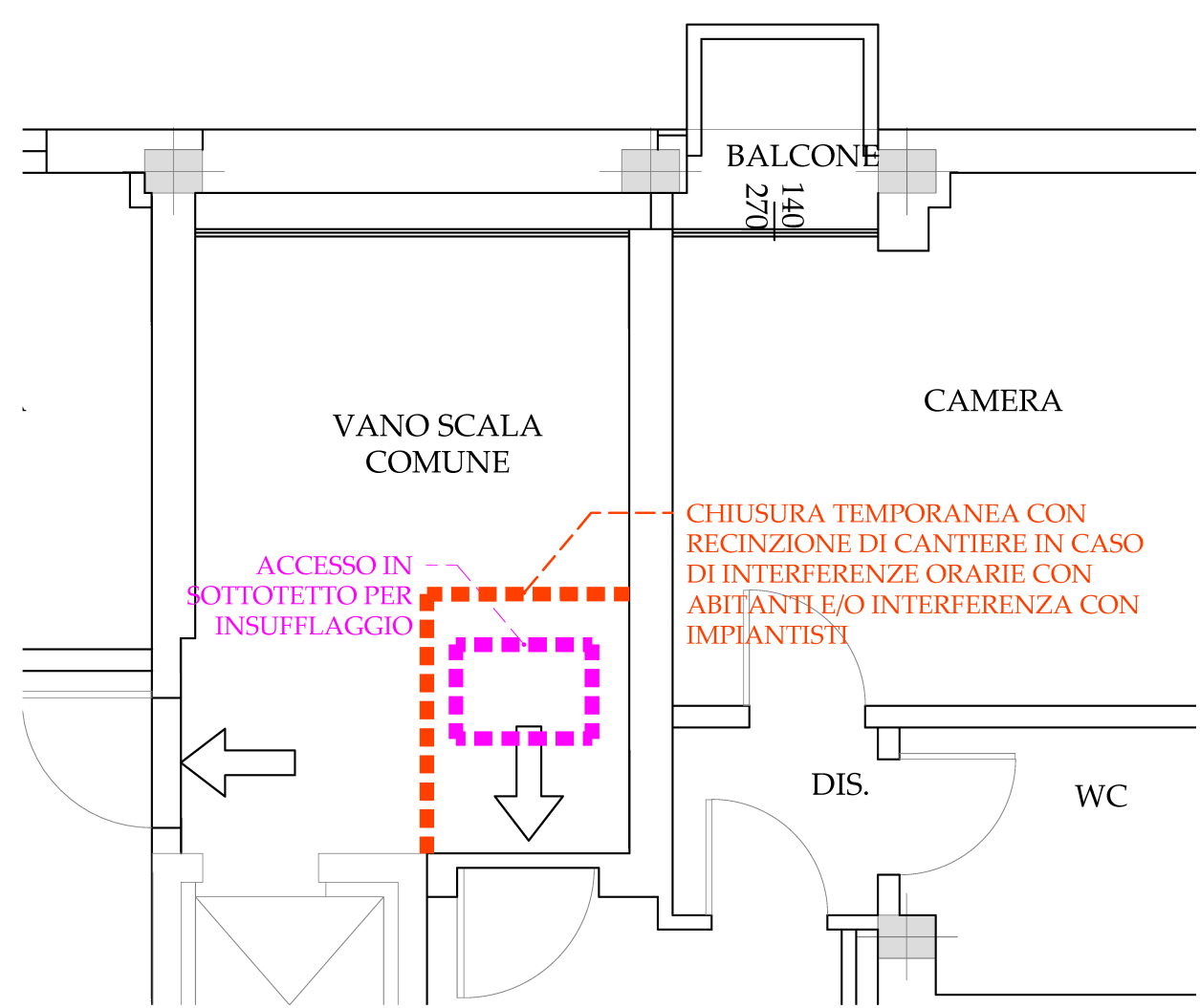
☺ SICUREZZA - Pianta secondo piano SCALA 1:50
